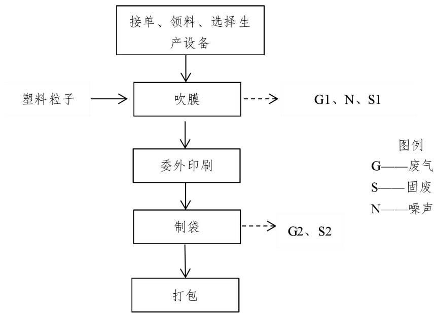
图 2-2 工艺流程及产污环节图
